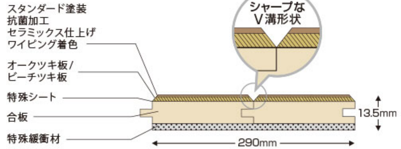
断面図(木口)
