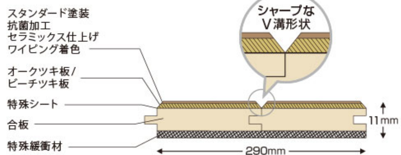
断面図(木口)
