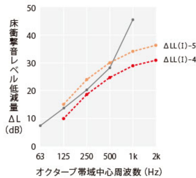
床衝撃音レベル低減量 試験結果
